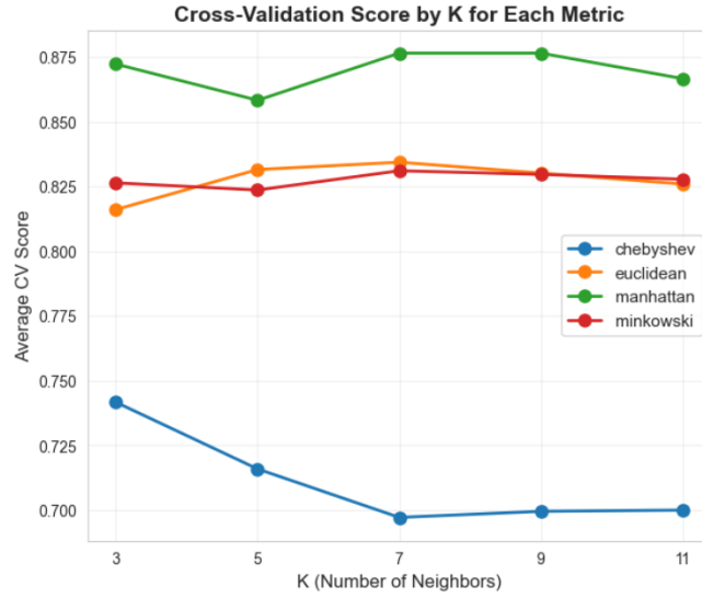
Fig. 2. Validation test with different parameter values
